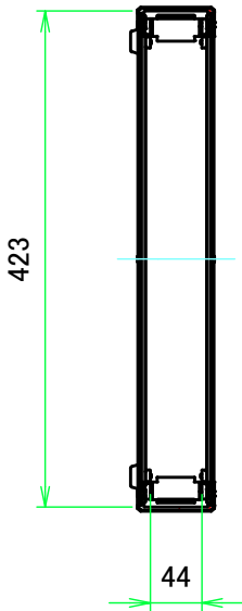
A-A ( 1:7 )
