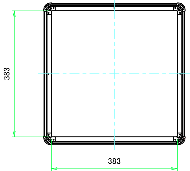
C-C ( 1:7 )
